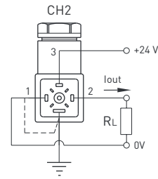
0-20mA or 4-20mA Output
